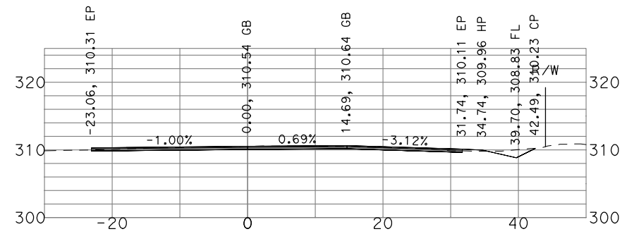
"GSB_R3_NB4" 541+00
