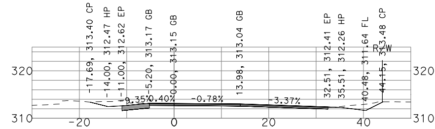
"GSB_R3_NB4" 461+00
