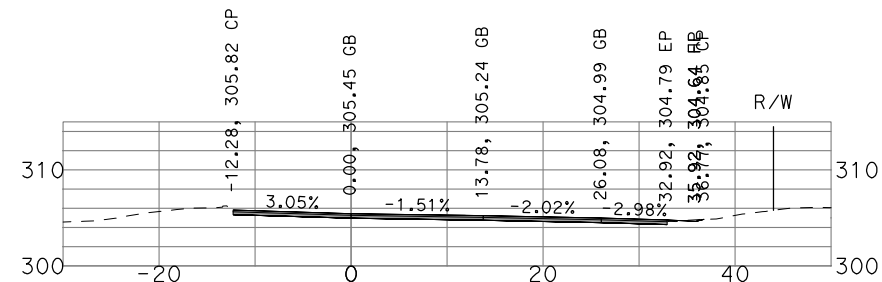
"GSB_R3_NB4" 492+00
