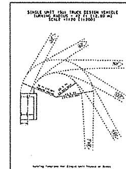
TRUCK TURN - TEMPLATE SCALE: NONE
